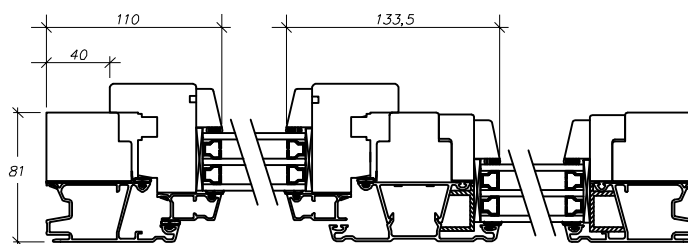
Öppningsbart fönster och fast del i samma karm
