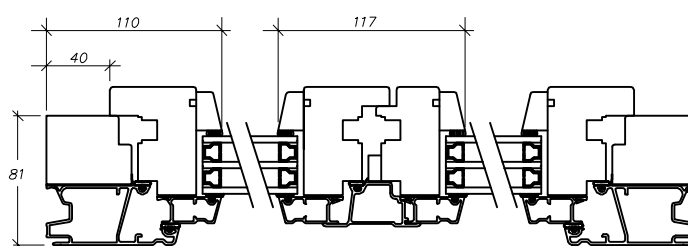
Tvåluftsfönster
