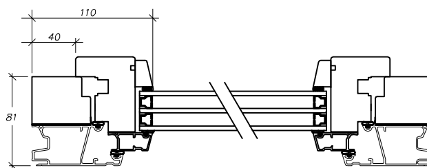
Enluftsfönster
